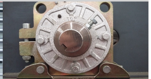
Inertia Brake
